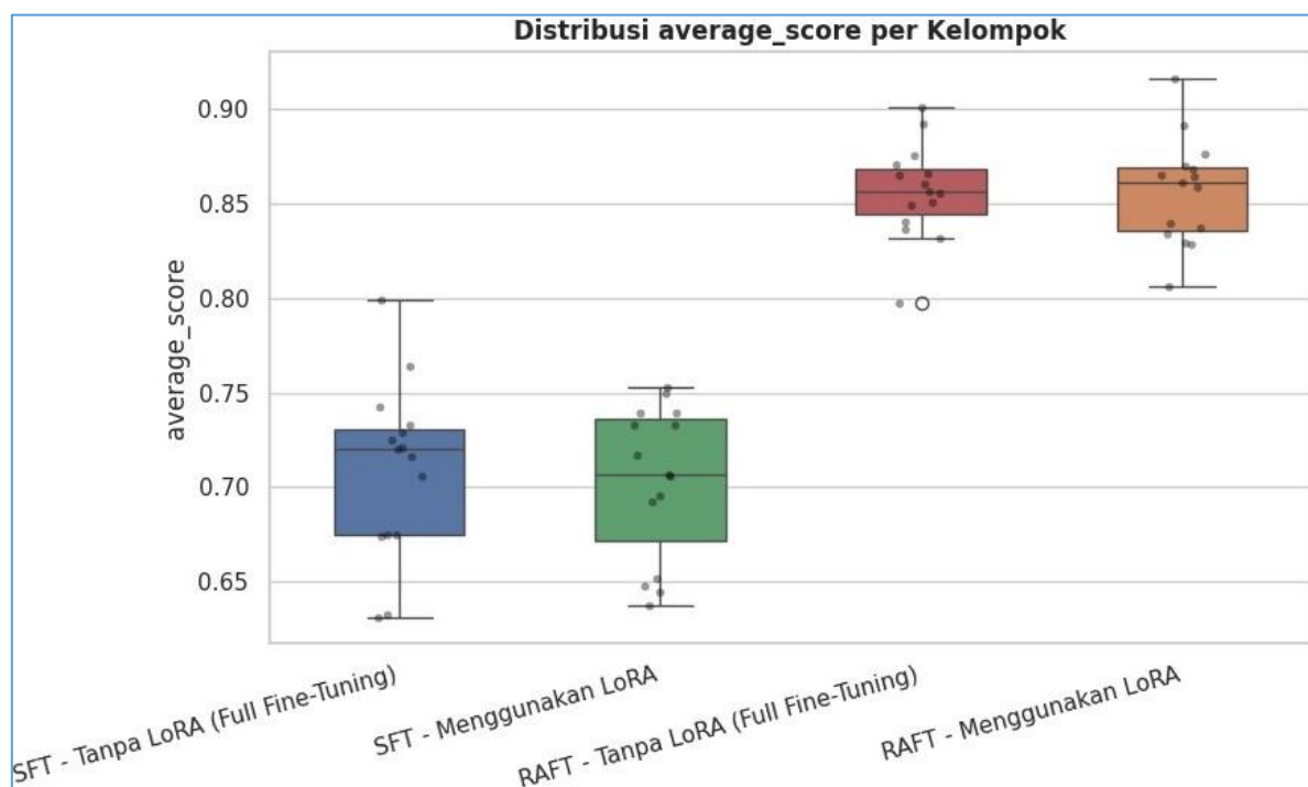
Gambar 4 Distribusi skor agregat pada 15 observasi per konfigurasi (3 epoch × 5 ukuran himpunan uji).
