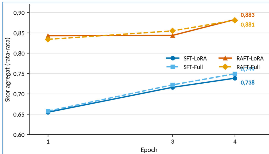
Gambar 3 Skor agregat per epoch (1, 3, dan 4) untuk empat konfigurasi.
