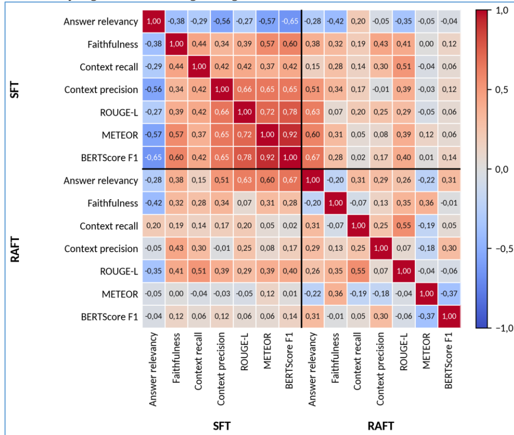
Gambar 5 Matriks korelasi antarmetrik leksikal, semantik, dan RAGAS
