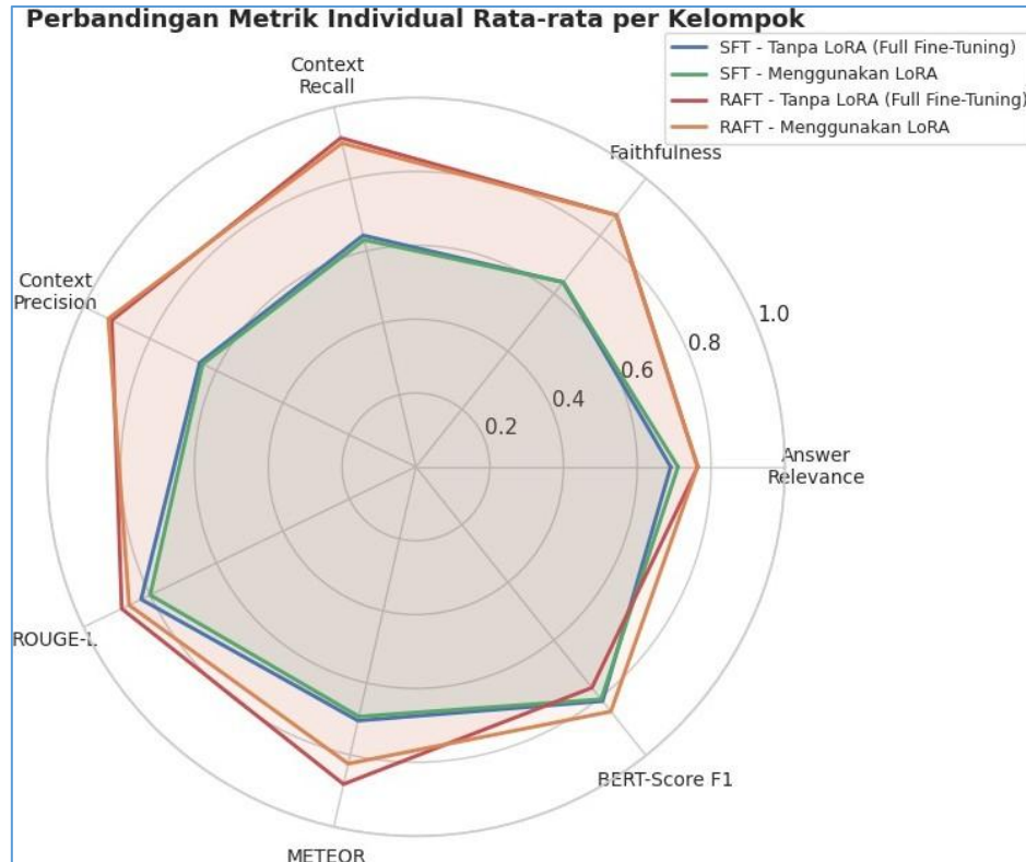
Gambar 2 Profil radar rata-rata tujuh metrik untuk empat konfigurasi.
