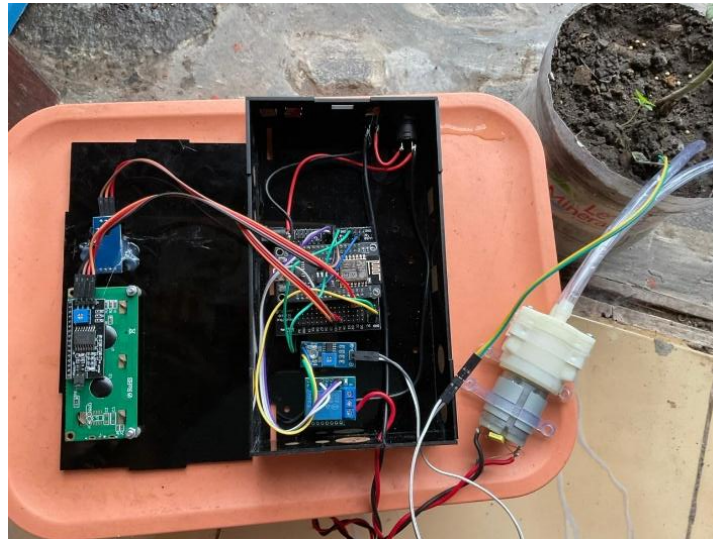
Gambar 4 Alat monitoring dan penyiraman otomatis
