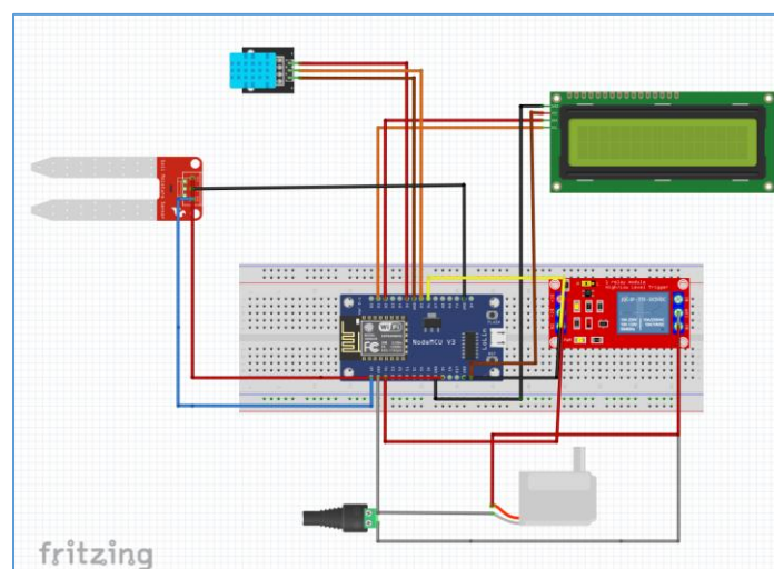
Gambar 3 memperlihatkan skema rangkaian sistem monitoring dan penyiraman otomatis tanaman tomat berbasis IoT.
