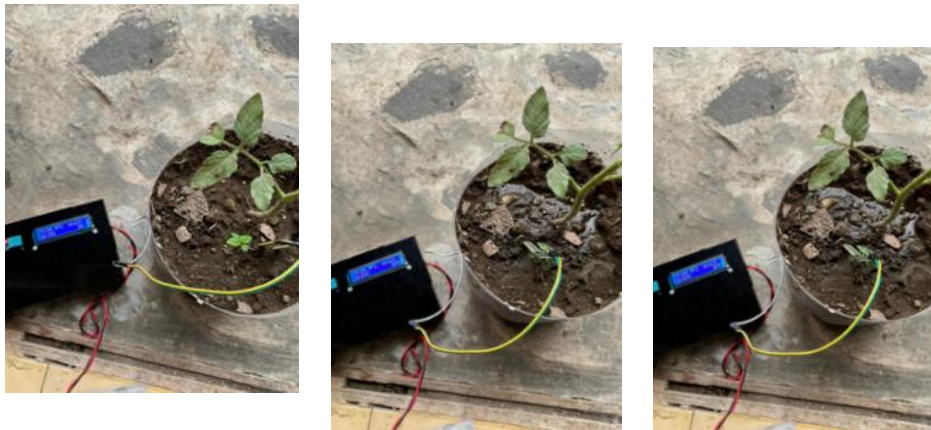
Gambar 5 Menampilkan proses pengujian sensor kelembapan tanah.
